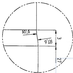
Detalj Y 4:1
