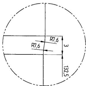
Detalj Y 4:1
